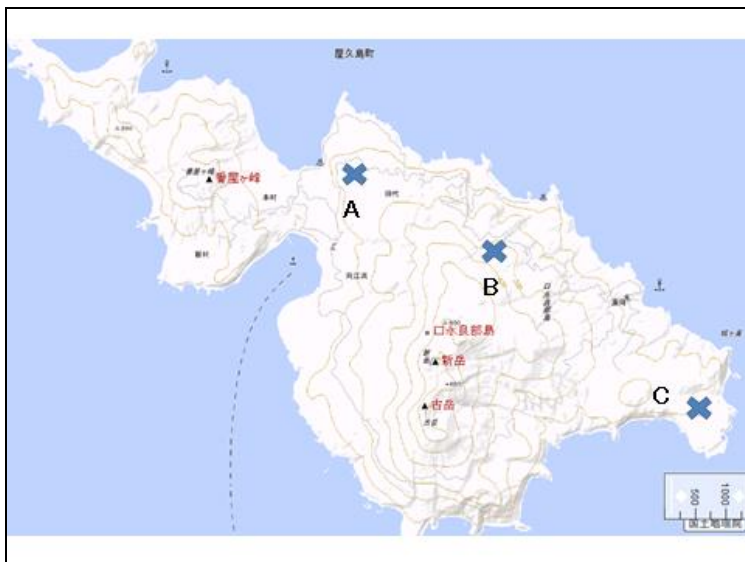
図5 ベルトトランセクトの設定箇所 A：十字・北、B：星ノ峰、C：女ヶ崎
